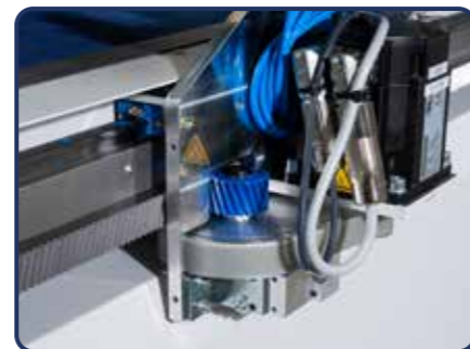
Zahnstangenantrieb für einen wartungsfreien und exakten Lauf der Brücke
